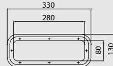
3号凸台 Base 3
