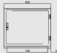
下面部分Lower portion
