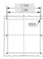
安装剖面 Installation section SK6621...
