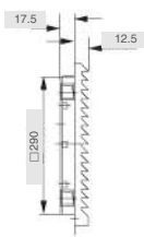
出口过滤器 Outlet filter SK6626. 300
