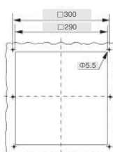
安装剖面 Installation section SK6626...
