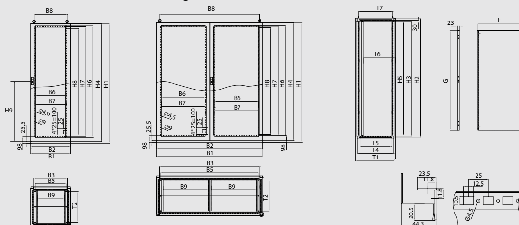
ES/BES系列细节图 ES/BES Series Detail Drawing
