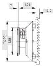
风扇及过滤器 Fan and filter SK6626. 230
