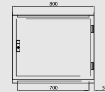
下面部分Lower portion
