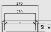
4号凸台 Base 4
