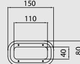
6号凸台 Base 6
