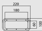
5号凸台 Base 5
